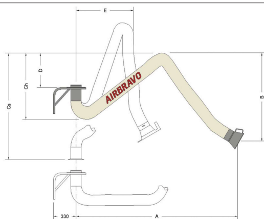
Montaggio pensile: con mensola a parete
